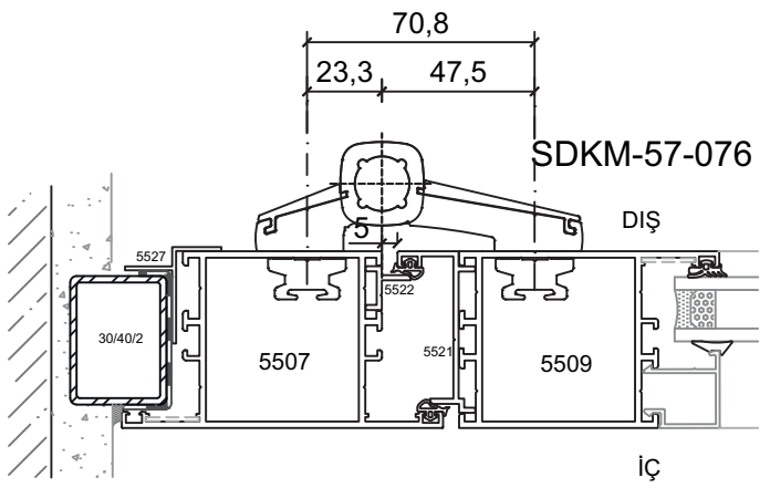
Kod : SDKM-57-076 Düz Kapazlama Mentеше ( 10 Adet / Paket )
