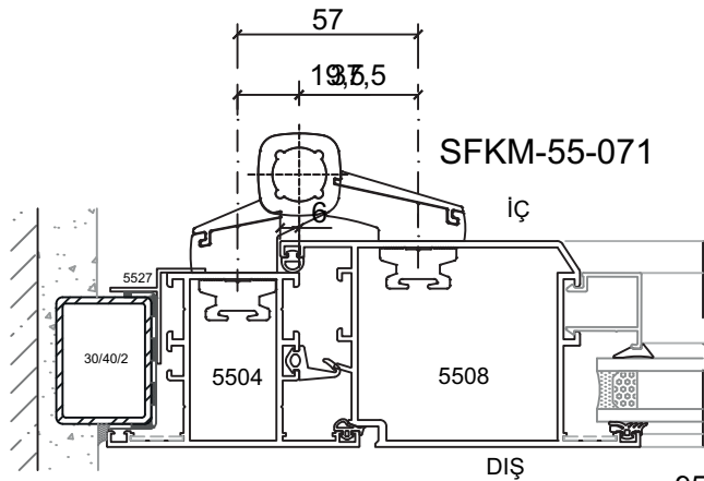
Kod : SFKM-55-071 Fugalı Kapazlama Mentеше ( 10 Adet / Paket )
